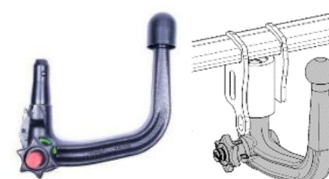
Vlečna kljuka, snemljiva brez orodja + 13-polni konektor
